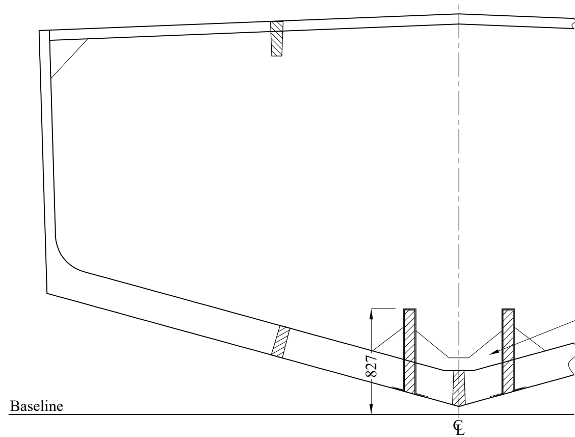
FR. 15
